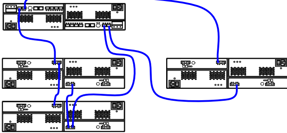
サンプル構成 (DS4700、EXP810 3台構成)
