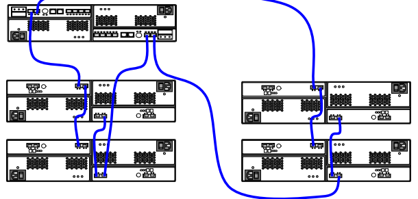
サンプル構成 (DS4700、EXP810 4台構成)
