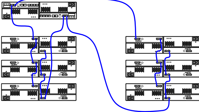
サンプル構成 (DS4700、EXP810 6台以上構成)
