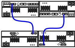
サンプル構成 (DS4700、EXP810 1台構成)
