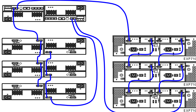
サンプル構成 (DS4700、EXP810とEXP710の混在構成)
