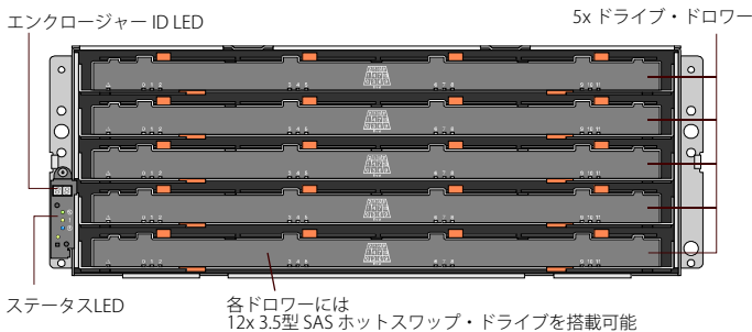
DM600S 4U60モデル・前面ビュー
