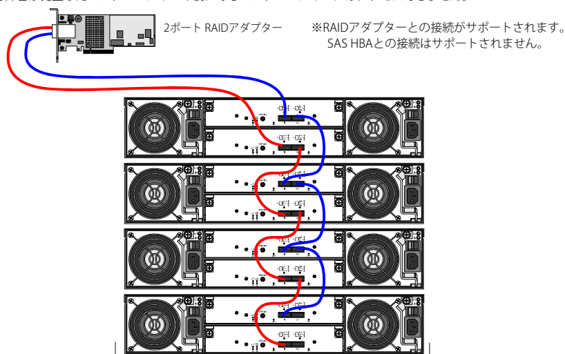
1RAIDアダプターにつき、最大4台までのエンクロージャーをデイジー・チェーン接続可能です。(E1012とE1024の混在可)
