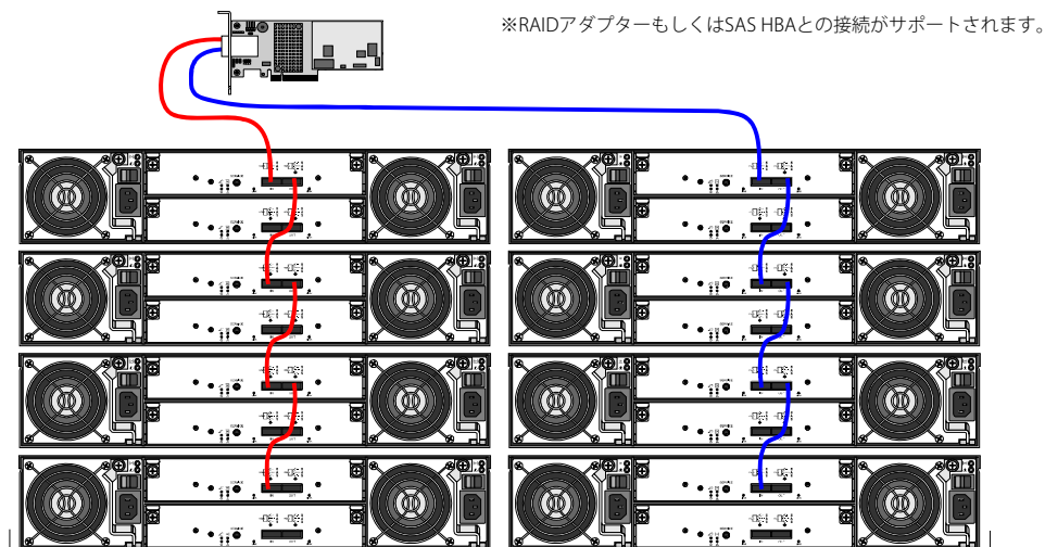
1アレイ・コントローラーにつき、最大8台までのエンクロージャーをデイジー・チェーン接続可能です。(E1012とE1024の混在可)
