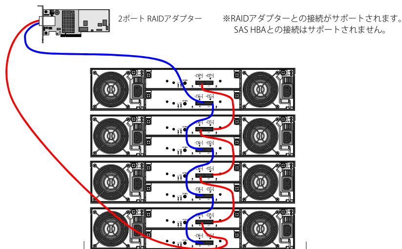
1RAIDアダプターにつき、最大4台までのエンクロージャーをデイジー・チェーン接続可能です。(E1012とE1024の混在可)
