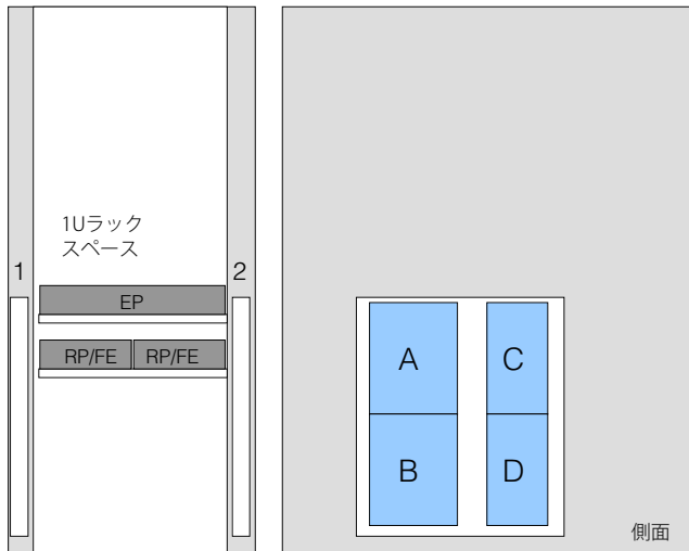
S2 25U スタンダード・ラック(93072RX/93072PX)
