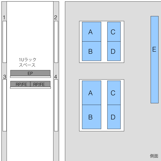
エンタープライズ 42U ラック (93084PX/93084EX)
