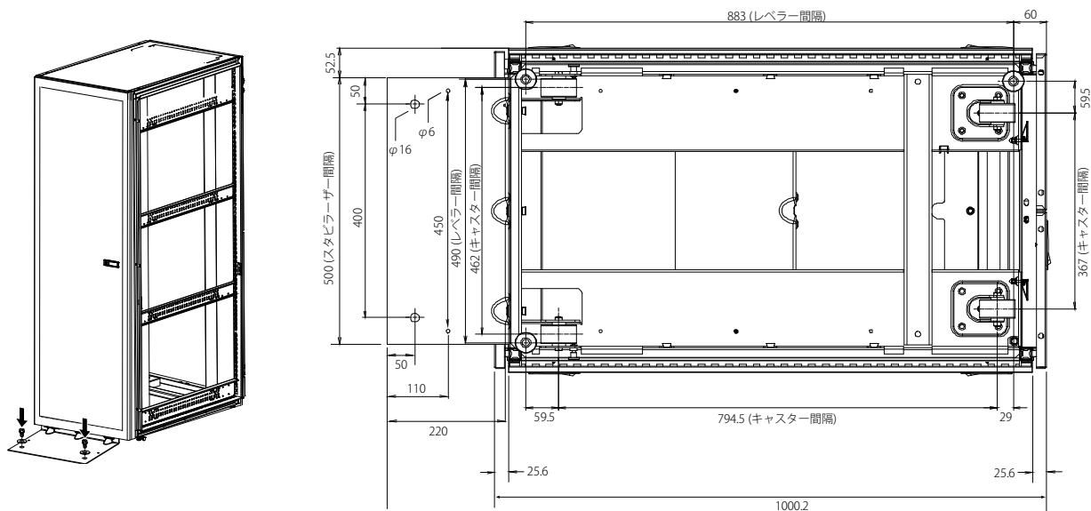
設置計画 (93074RX/93074XX/93614PX/93614EX) (S2 25U スタンダード・ラック(93072RX/93072PX)共通)
