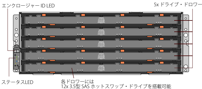
DM600S 4U60モデル・前面ビュー
