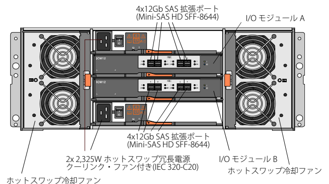
DM600S 4U60 インターフェイス・背面ビュー
