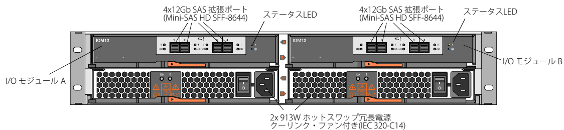
DM120S インターフェイス・背面ビュー
